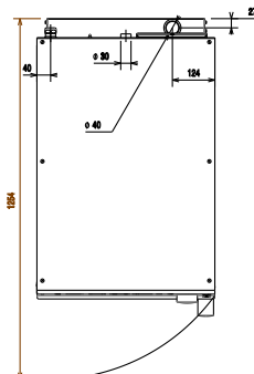
Boven aanzicht
