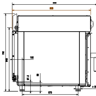
Zij aanzicht
